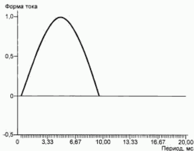
Рисунок А.2 — Форма тока при однополупериодном выпрямлении
